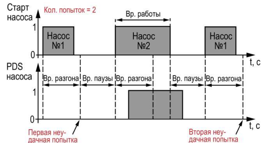
Рисунок 14.8 – Перезапуск насоса
