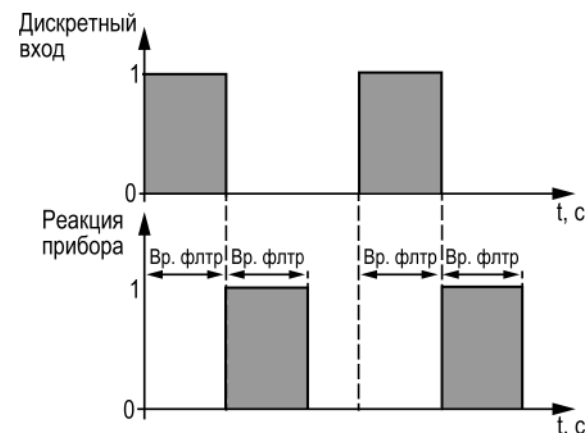
Рисунок 11.5 – Принцип работы времени фильтрации
