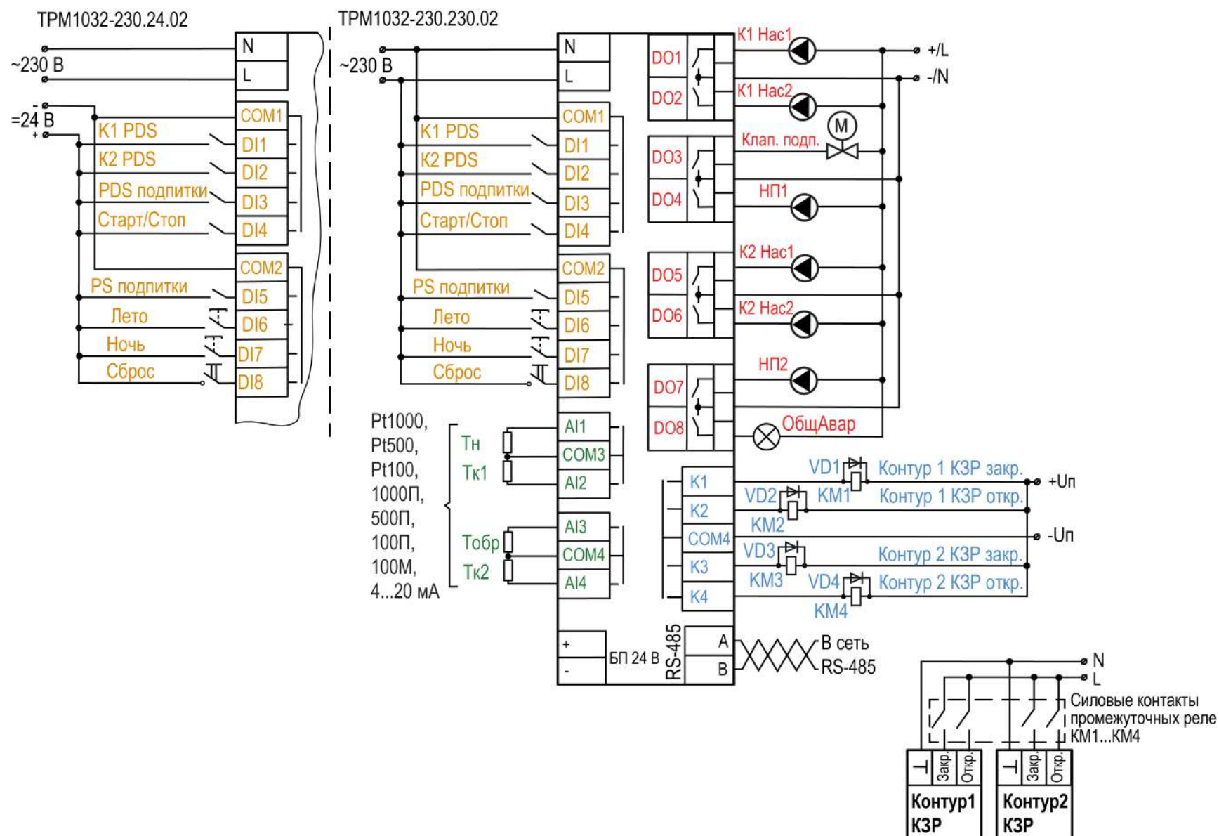
Рисунок 9.3 – Схема подключения
